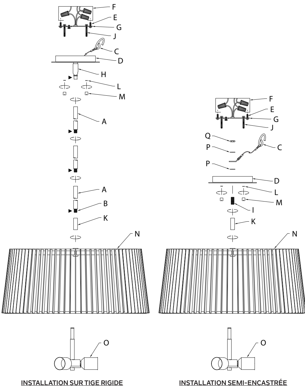
INSTALLATION SUR TIGE RIGIDE
